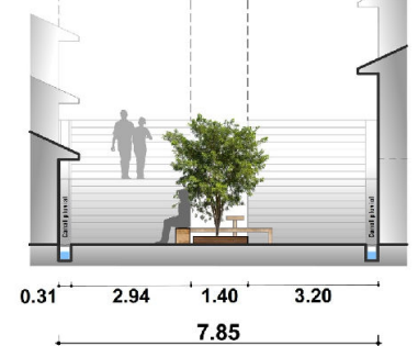
PASAJE C PLANTA Y SECCION G-G Via peatonal
