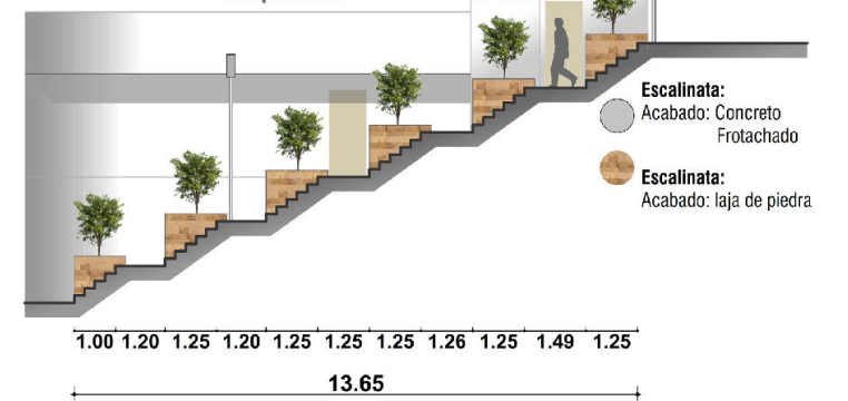
PASAJE C PLANTA Y SECCION G-G Via peatonal
