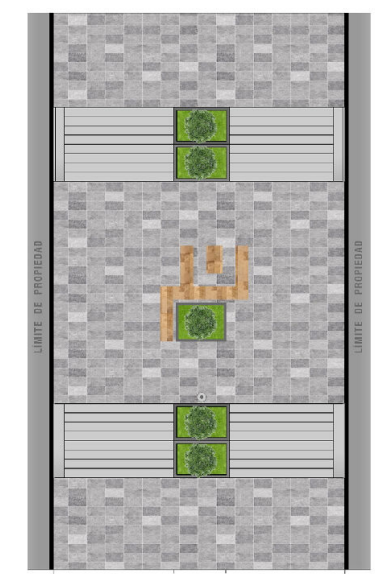
PASAJE 3 PLANTA Y SECCION E-E Via peatonal
