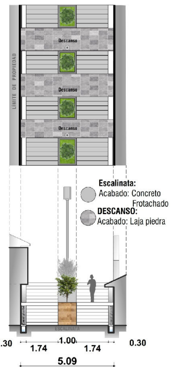
PASAJE C PLANTA Y SECCION F-F Via peatonal
